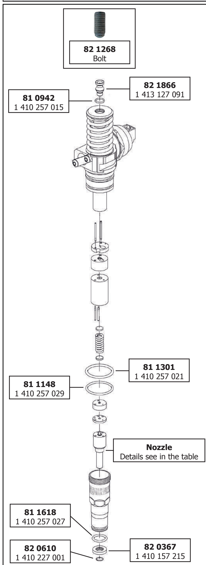
Unit Injector (UIS/PDE) Typ 5
