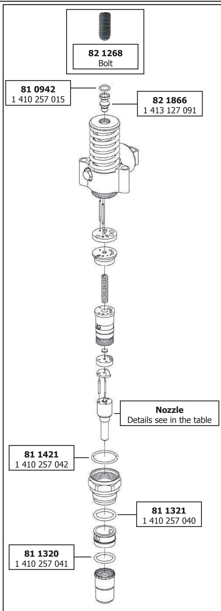
Unit Injector (UIS/PDE) Typ 6
