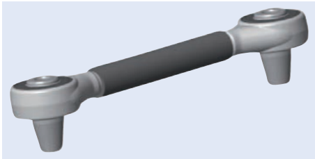
LEMFÖRDER Transverse link Pipe Ø 36 mm
